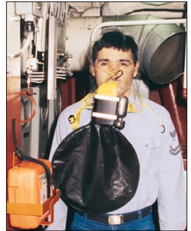
L'EEBD Ocenco M-20.2 montré est prêt à être utilisé pour l'évacuation.
